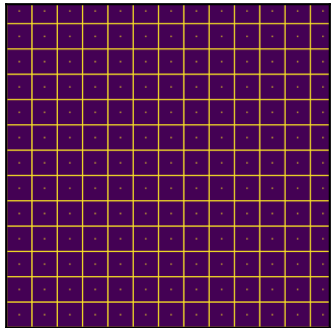
Input array
